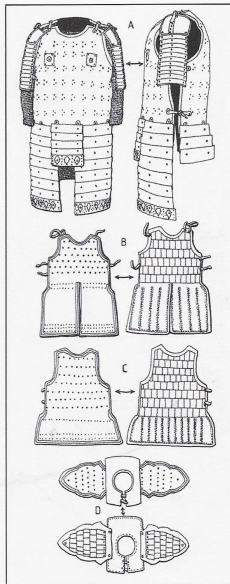
Armadura de finales del siglo XIV, como las que llevaban la Horda de Oro y las tropas de Timur. A: armadura ensamblada vista de frente y de lado. B a D: exterior e interior de la parte trasera (B), la parte delantera (C) y el hombro (D). (Reconstrucción realizada por el Dr. M. Gorelik y L.A. Parusnikov de la Academia de Ciencias de Moscú. La armadura se encuentra ahora en el Museo del Campo de Batalla de Kulikovo).
